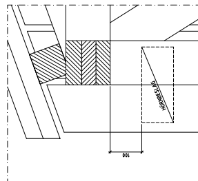
HÖRNBESLAG TYP 2
