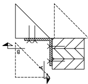
HÖRNBESLAG TYP 2
