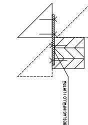
HÖRNBESLAG TYP 3
