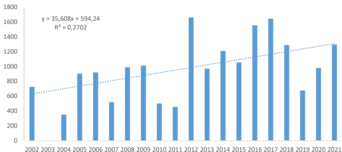
Figur 2. Antall sædgjess på myteplassen i Vestre Jakobselv på Varangerhalvøya i årene 2002-2021.
