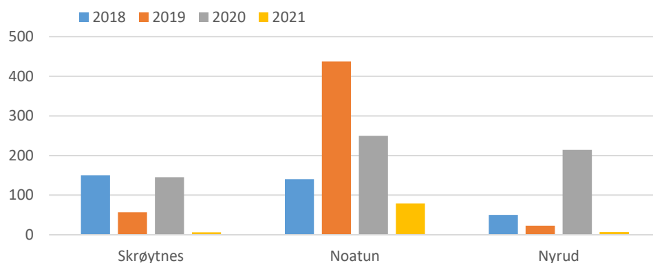
Figur 4. Fordeling av sædgås i Pasvik i årene 2018-2021.
