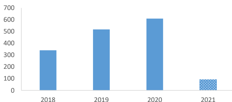
Figur 3. Totalt antall skogssædgjess talt i Pasvikdalføret under vårrasting i årene 2018-2021. Året 2021 er skravert da det reelle antall taigasædgjess ikke ble talt da forekomsten var på sitt høyeste.
