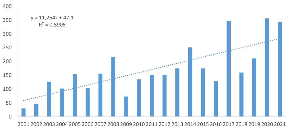
Figur 1. Årlig største antall observerte sædgjess på Valdakmyra under vår-rastingen i årene 2001-2021.
