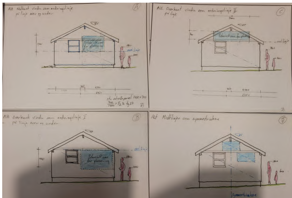
Figur 2.2. Søkers skisser av alternative plasseringer for solcellepanelene. Sendt til forvalter 28.10.2025.
