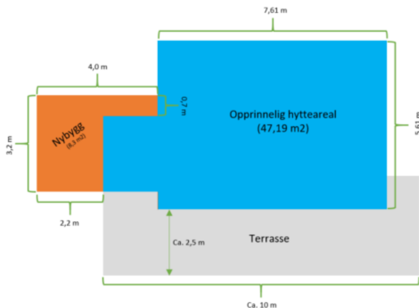
Fig. 1. Planløsning som viser omsøkt tilbygg (oransje).
