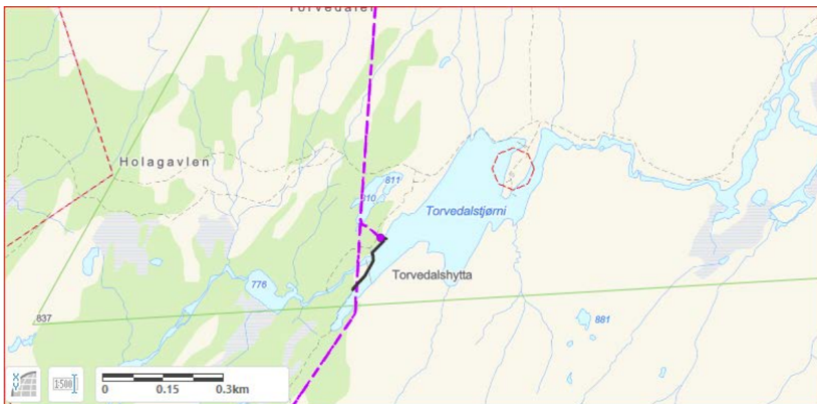
Figur 2 Torvedalstjøerni ligger innanfor Stølsheimen Landskapsvernområdet (grønn linje): Rød linje til venstre er kommunegrensa mellom Vaksdal og Voss. Stiplet linje (lilla farge) er driftstunnelen til Evanger kraftverk og svart linje er dammen ved utløpet av Torvedalstjøerni.
