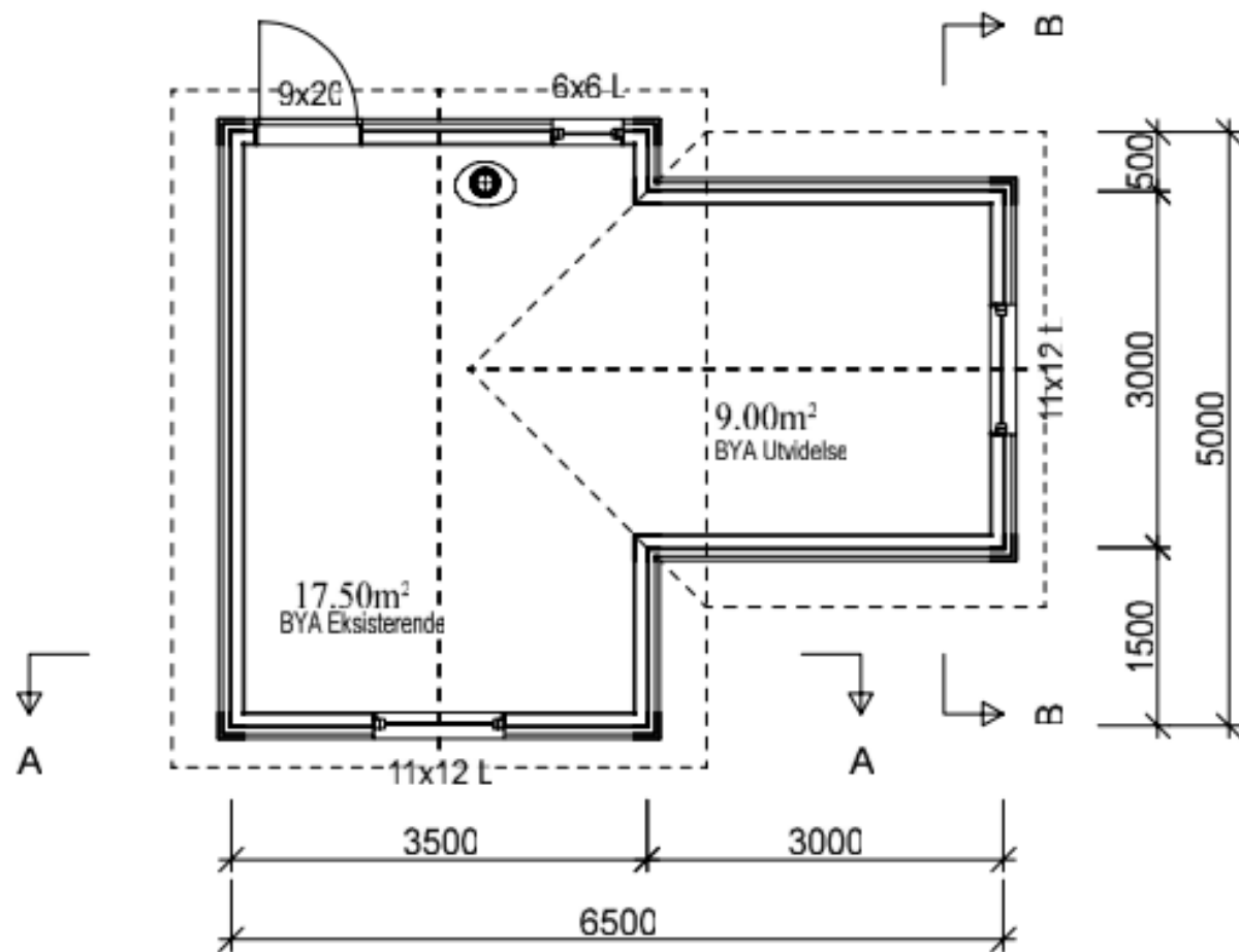
Forstørring av tegning fra plantegning for fremvisning av dimensjoner – del 2.
