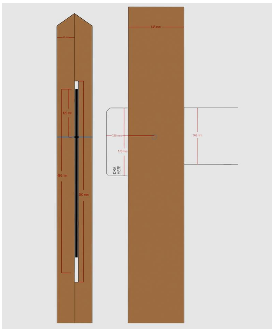
Skisse av stolpe for natursti (Kilde: designmanualen for Norges nasjonalparker)
