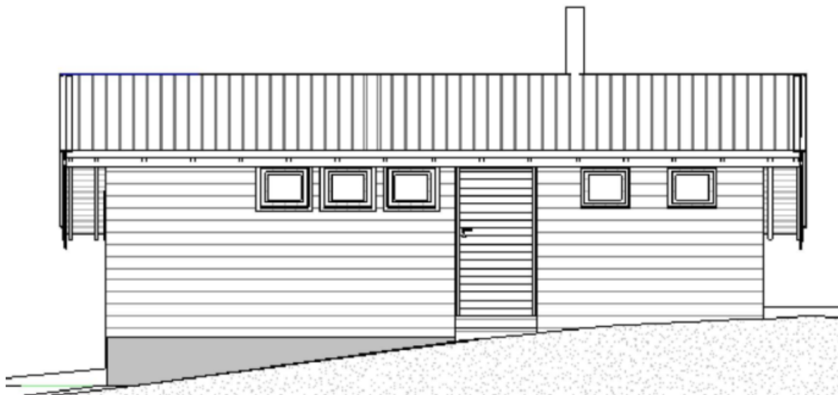
Eksisterende og ny fasade på vestvegg
