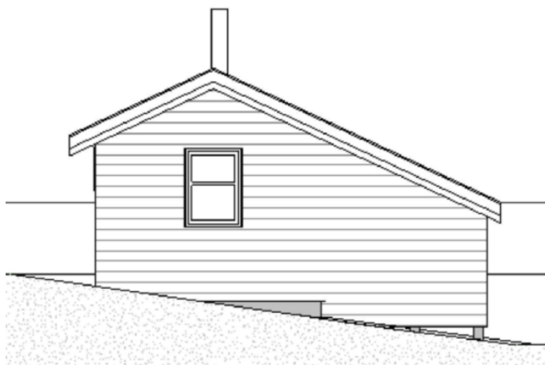
Fasadeendring av vestvegg på hovudhytta
