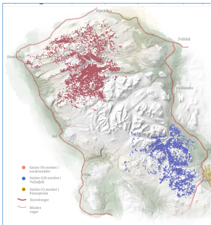
Figur 3. Kartplott – posisjonsdata fra GPS-merkede simler i perioden desember-mars årene 2009-18.
