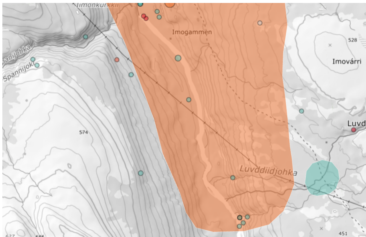
Figur 1: Kartutdrag fra Artsdatabanken. Rød markering er leveområde for Tretåspett og blått område er leveområde for dvergfolk
