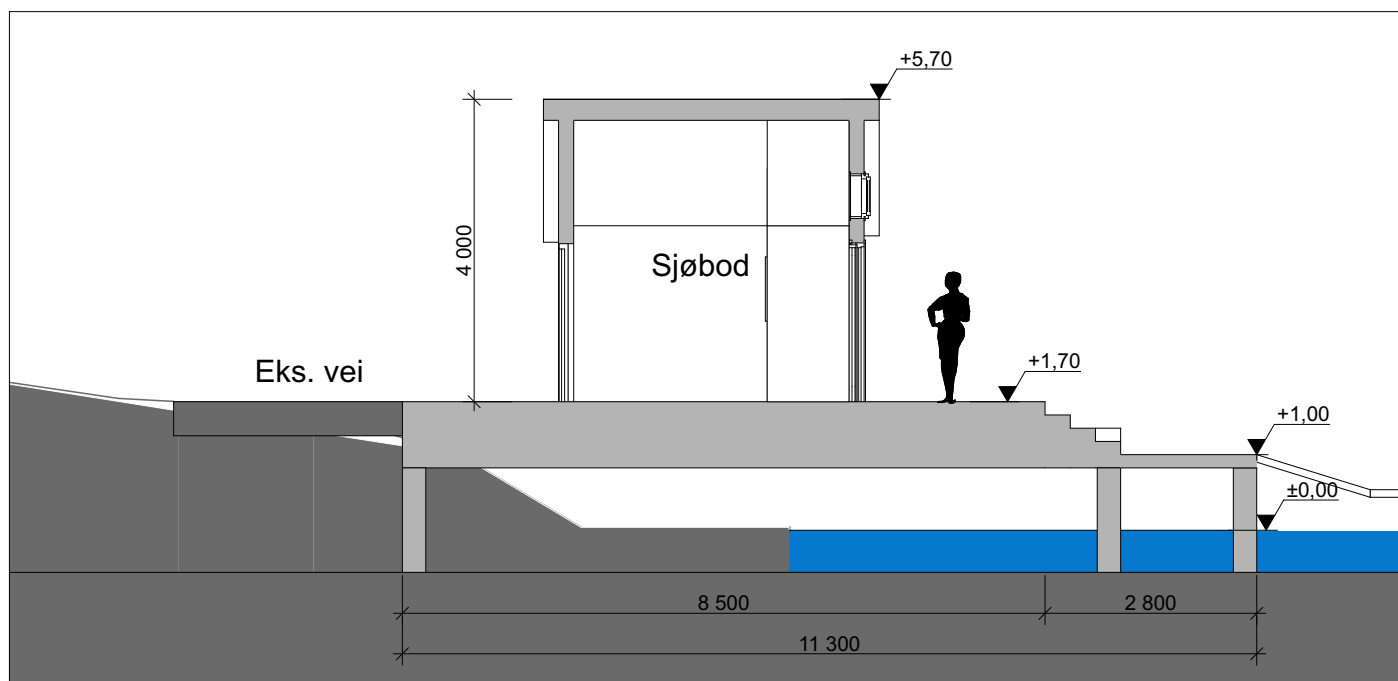
Snitt B
