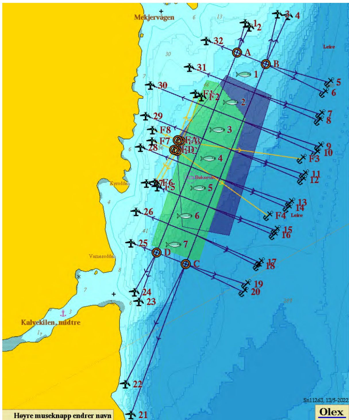
Figur 3. Anlegg og flåte med tilhørende fortøyningslinjer. Grønt skravert område er område som vi ligger på i dag. Lilla skravert område er avsatt akvakulturområde i kystsoneplanen.
