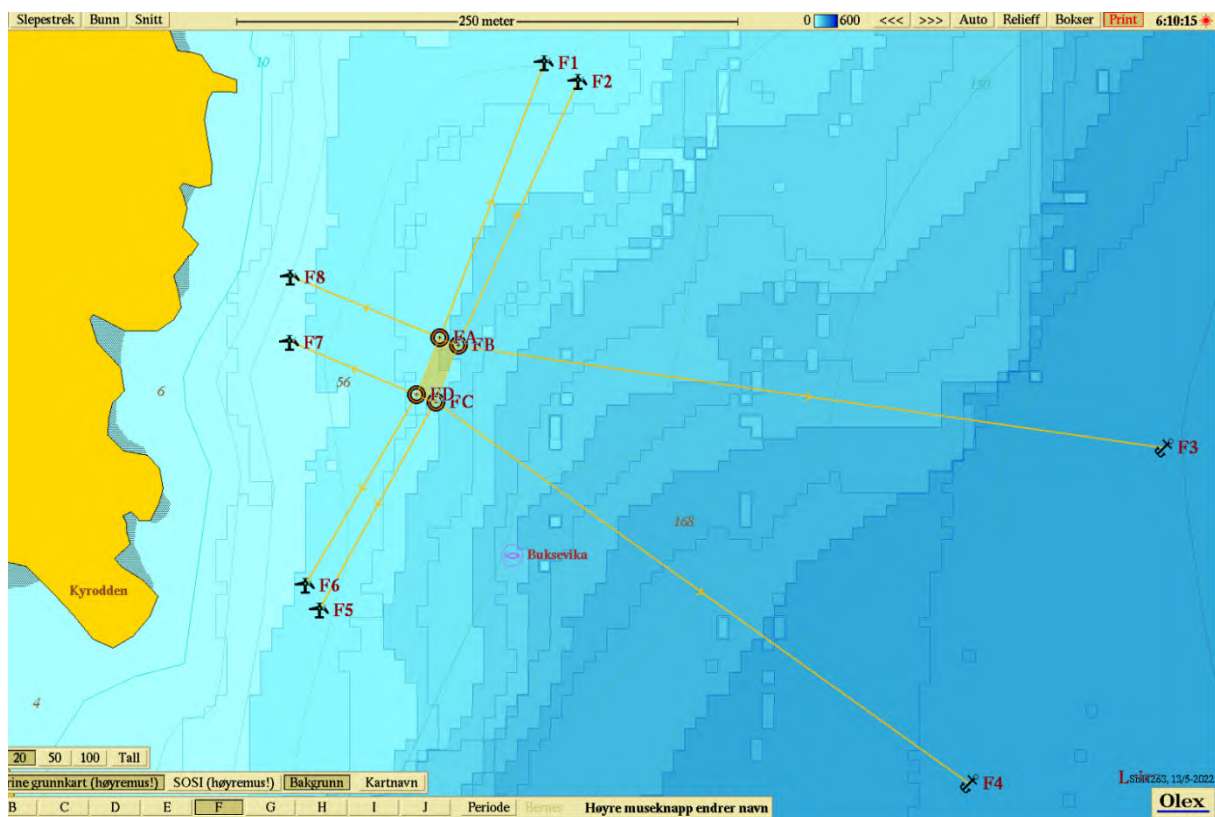
Figur 1. Flåte med tilhørende fortøyningslinjer
