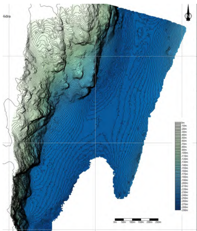
Figur 3. Backscatter-kart som viser relativ hardhet i området. Bunnkartlegging utført av ROV AS 20.03.18. Fargekoder for hardhetsskala i øvre høyre hjørne.
