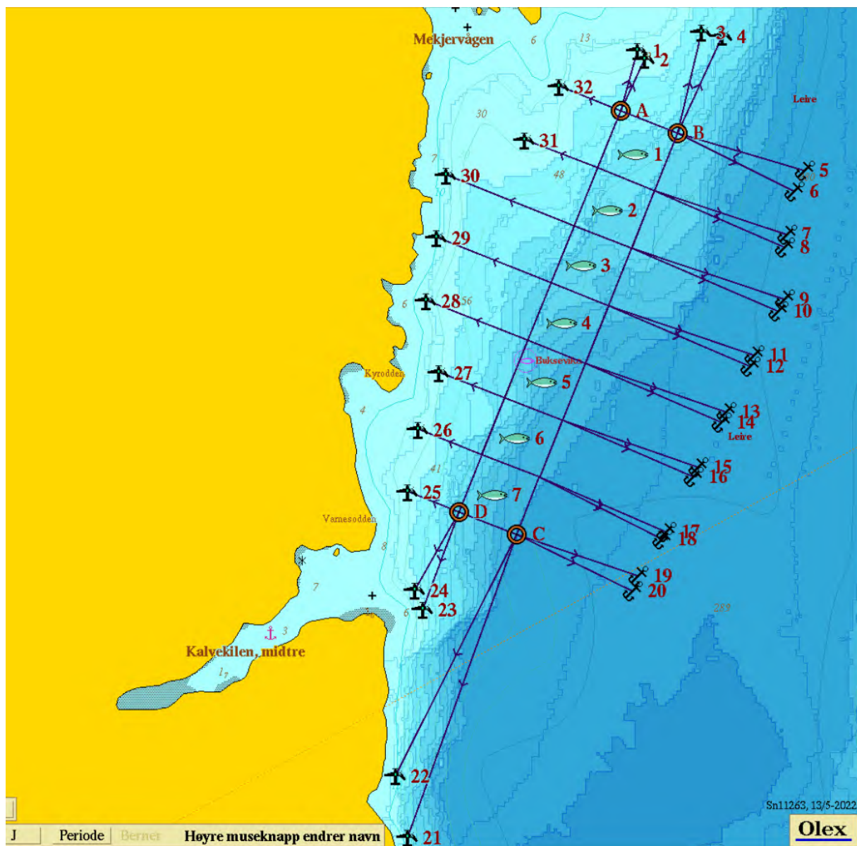
Figur 2. Anlegg med tilhørende fortøyningslinjer.
