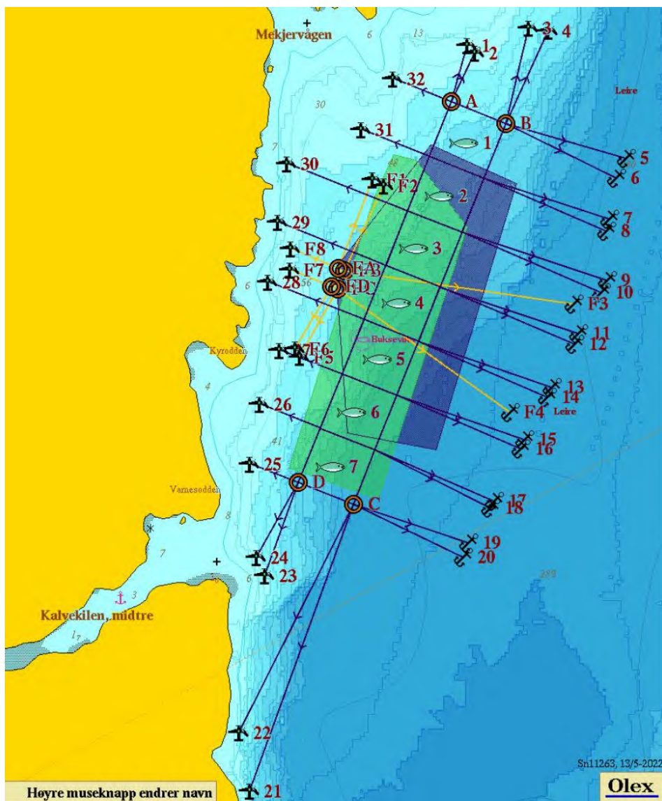
Figur 2. Anlegg og flåte med tilhørende fortøyningslinjer. Grønt skravert område er område som vi ligger på i dag. Lilla skravert område er avsatt akvakulturområde i kystsoneplanen.
