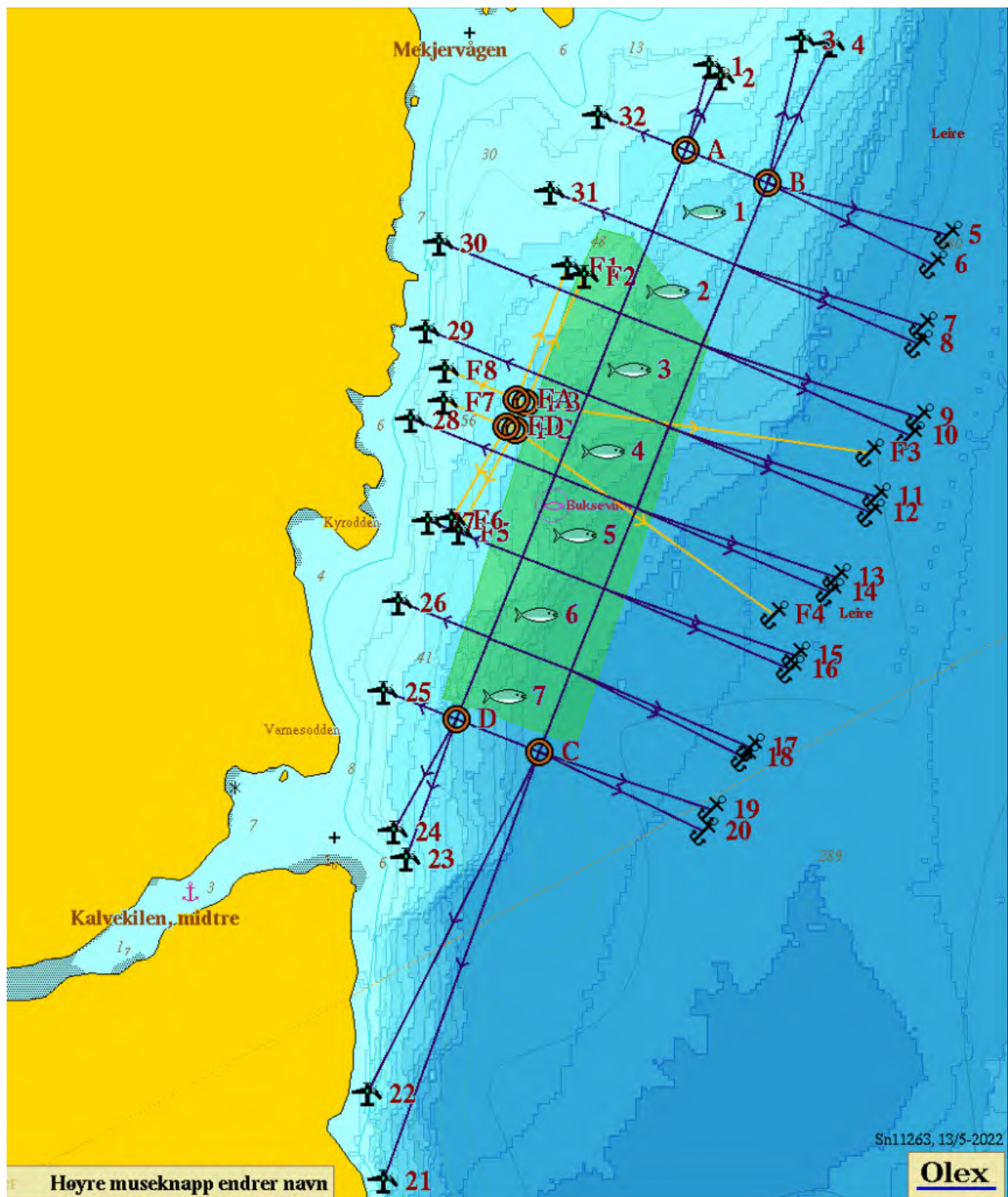
Figur 5. Anlegg og flåte med tilhørende fortøyningslinjer. Grønt skravert område er område som vi ligger på i dag.
