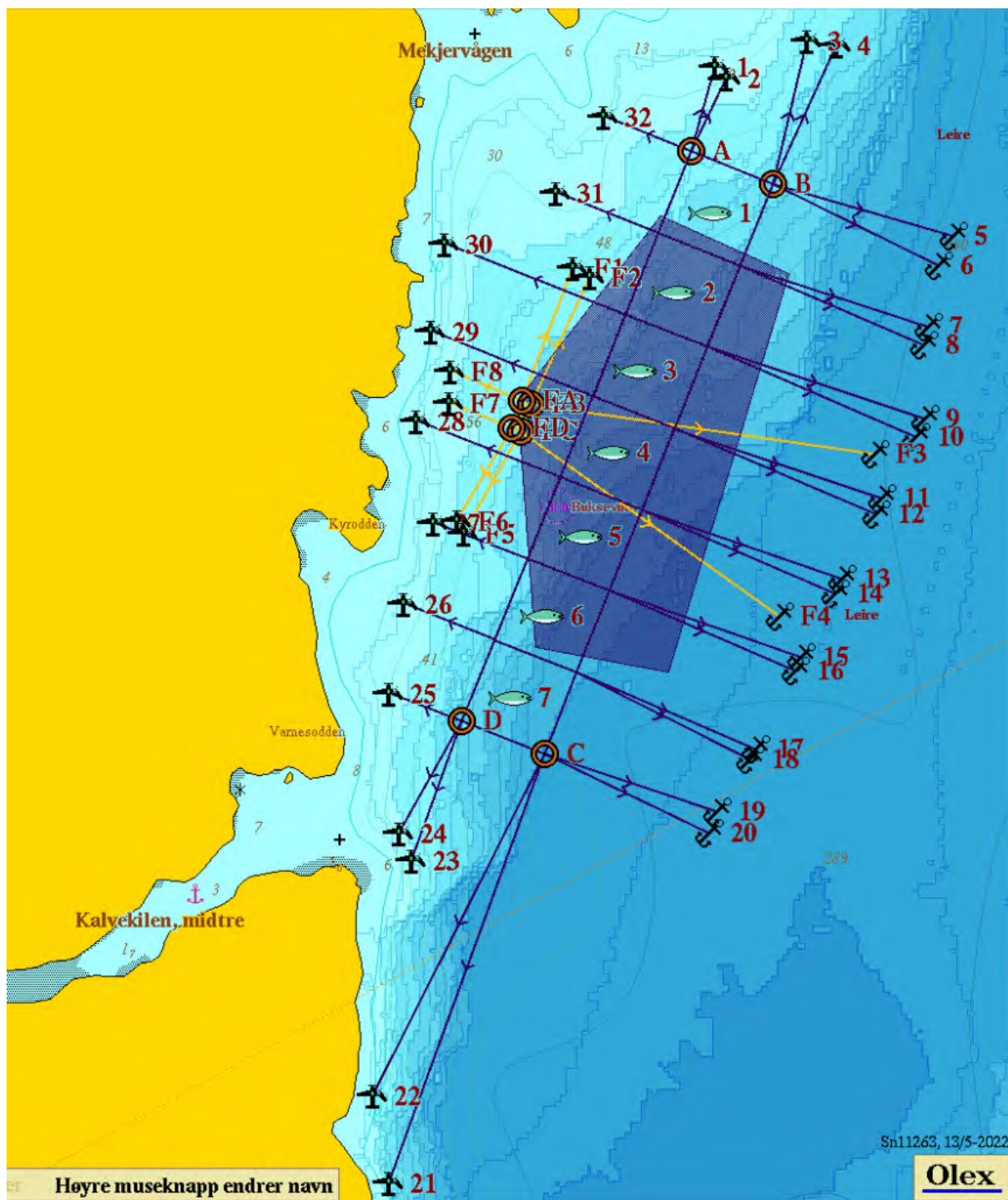
Figur 4. Anlegg og flåte med tilhørende fortøyningslinjer. Lilla skravert område er avsatt akvakulturområde i kystsoneplanen.
