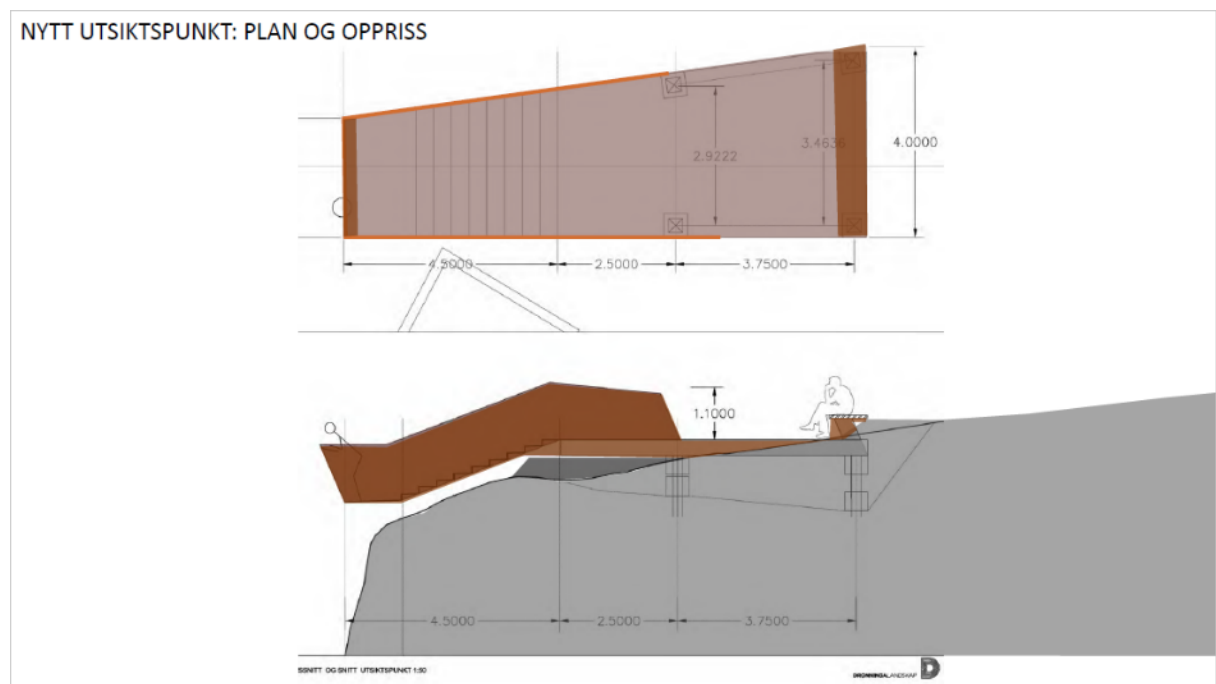
Figur 5: Plan og oppriss
