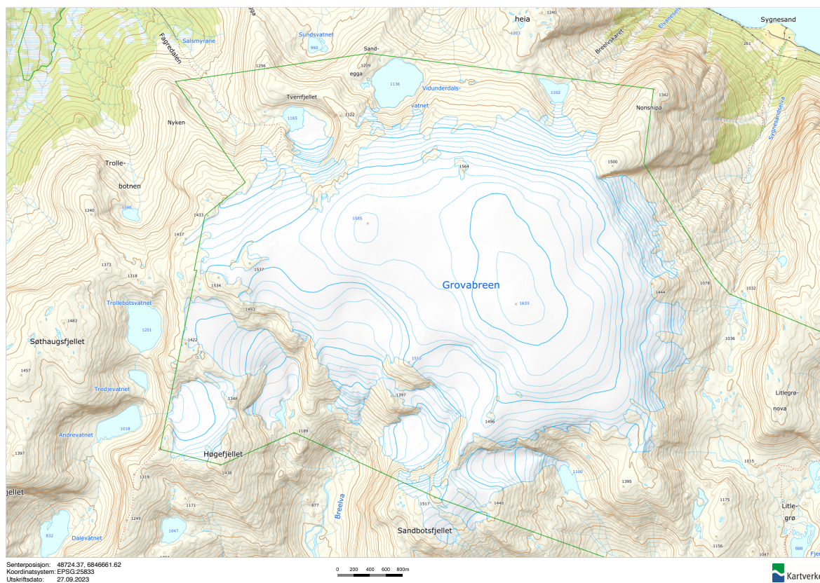
Figur 3.13.1 Topografisk kart over Grovabreen og områda rundt. Den grøne streken markerer grensa for nasjonalparken. Kart: norgeskart.no.
