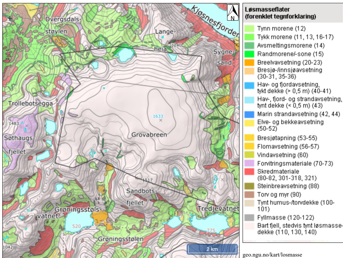
Figur 3.13.2 Lausmassekart over Grovabreen og områda rundt.
