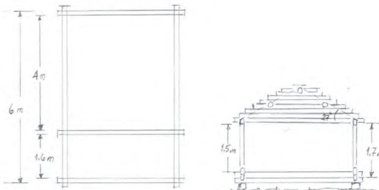
Plan- og snitt- tegninger.
