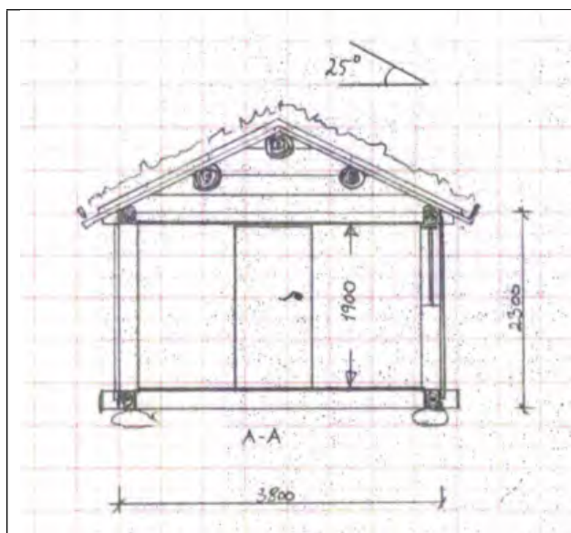
Målsatt plantegning som følger søknaden, jf. saksdokument 1.
