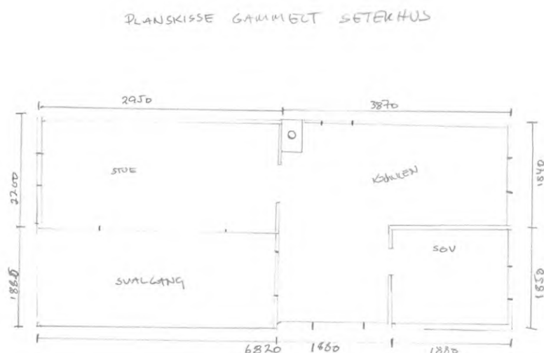
Figur 1: planskisse gammelt seterhus
