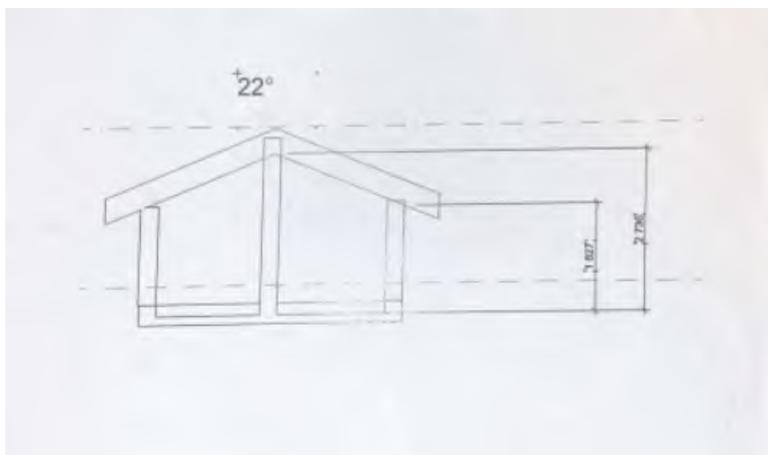
Figur 4: Snitt, mål angitt i figur: gesimshøyde under vindskie: 1,827. Rafthøyde: 2,736.
