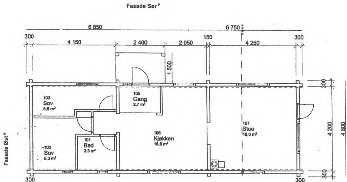
Figur 5: Planskisse over nytt seterhus
