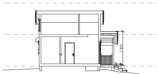
1:100 Snitt A
