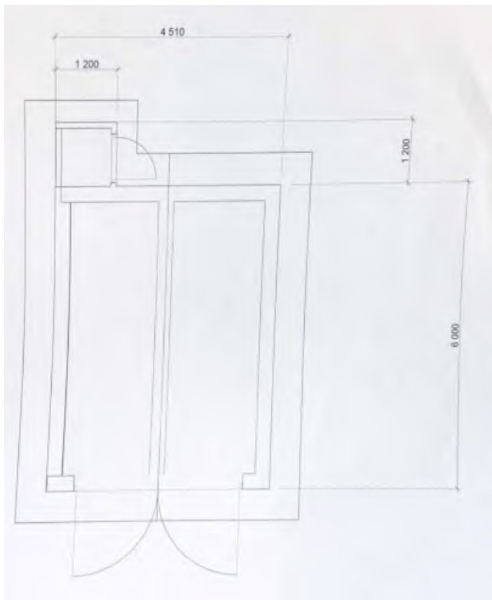
Figur 3: Planskisse. Naust med plass til to båter, samt utedo.
