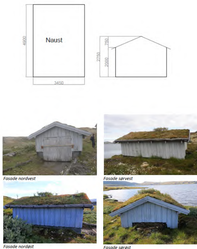
Figur 8: Oppmålt naust (16,9 m 2 BYA).
