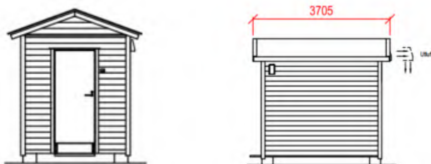
Byggetegninger - fasader – front og side
