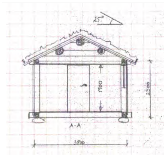
Målsatt plantegning som følger søknaden, jf. saksdokument 1.
