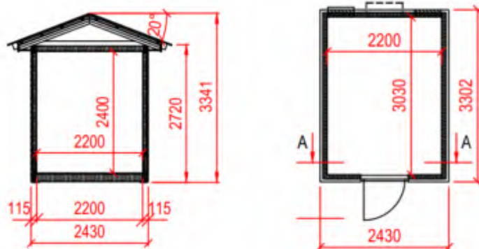
Byggetegninger – snitt og plan
