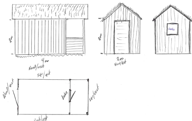
t.h: skisse av nytt vedskjul (erstatte eksisterende)
