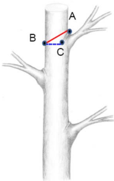
Figur 4.1.12. Prinsippskisse for kronereduksjonssnitt. Det skal skjerast tilbake slik at greina har ein diameter på minimum 1/3 av diameteren til stammen. Snittet skal leggjast frå toppen av borkåsen (pkt. A) og førast diagonalt på skrå ned mot pkt. B. Ein finn pkt. B ved å trekkje ei linje frå botnen av borkåsen (C) og vassrett på stammen. Illustrasjon frå Kjersti Wilhelmsen; Beste praksis for nedskjering av tre. Norsk Trepleieforum.
