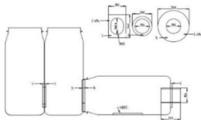
Teknisk tegning av fjellrevautomatene, se også foto under.
