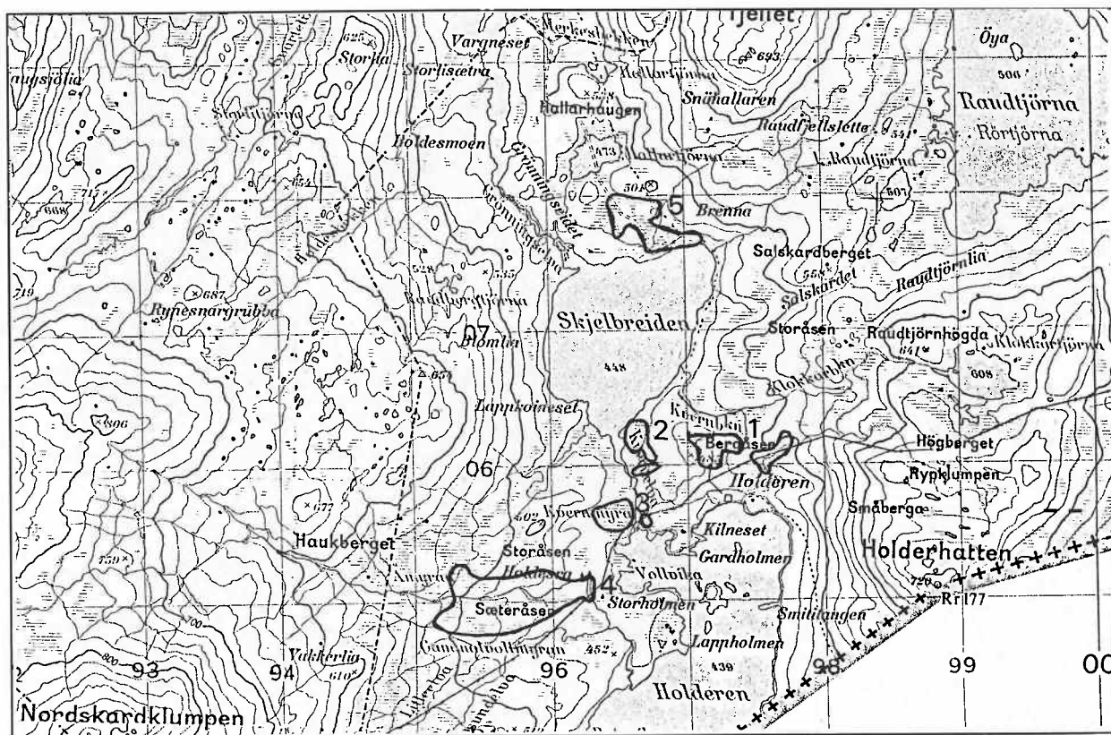
Figur 5. Holderen i Snåsa kommune. Utsnitt av kartblad 1823 II (M711), målestokk 1 : 50 000. Fem lokaliteter er avmerket på kartet.
