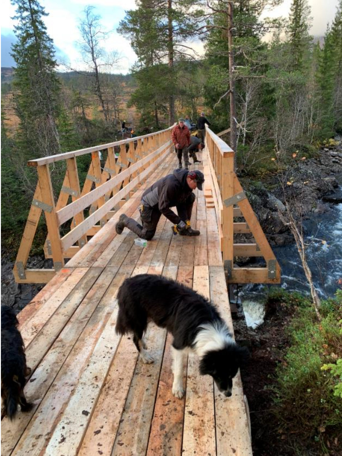
Fig. 1: Bru over Skjækra ferdigstilt høsten 2020. Finansiert av nasjonalparkstyret ved hjelp av tiltaksmidler og bygd av Harbakvollen seterlag.
