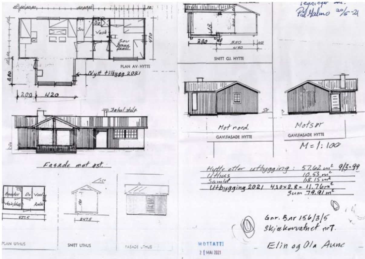
Fig. 1 Tegninger av Skjækervatnet 7, Gnr/Bnr/Fnr 156/3/5
