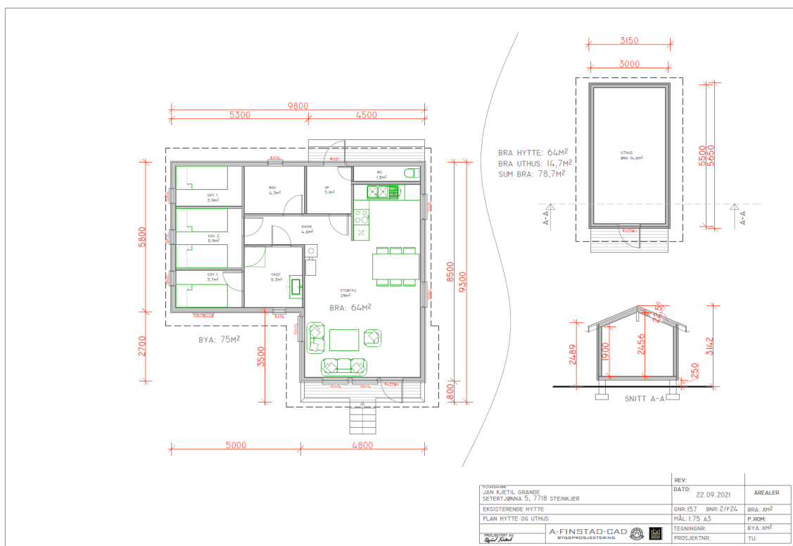
Fig. 2: Tegninger av nytt uthus og eksisterende hytte Setertjønna 5 i Steinkjer kommune
