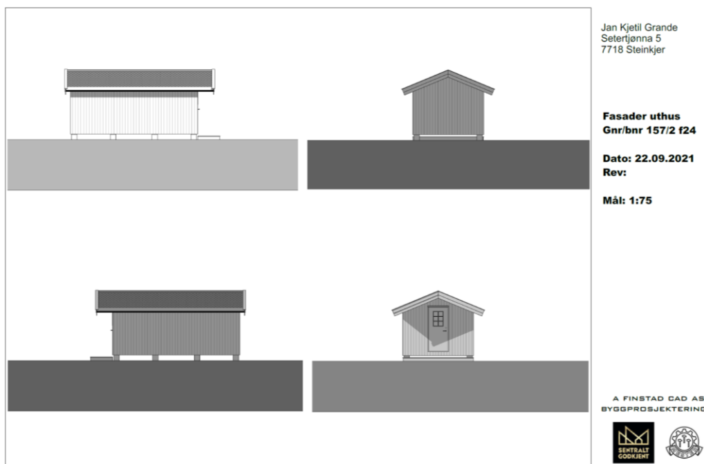
Fig. 3: Fasadetegninger av nytt uthus ved hytte Setertjønna 5 i Steinkjer kommune
