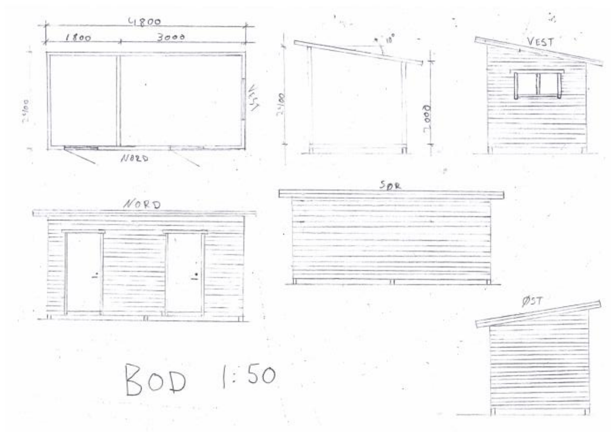
Fig. 1: Tegninger over omsøkt uthus til gjeterhytte ved Hykla, sommerboplassen til Låarte sijte i Lierne kommune.
