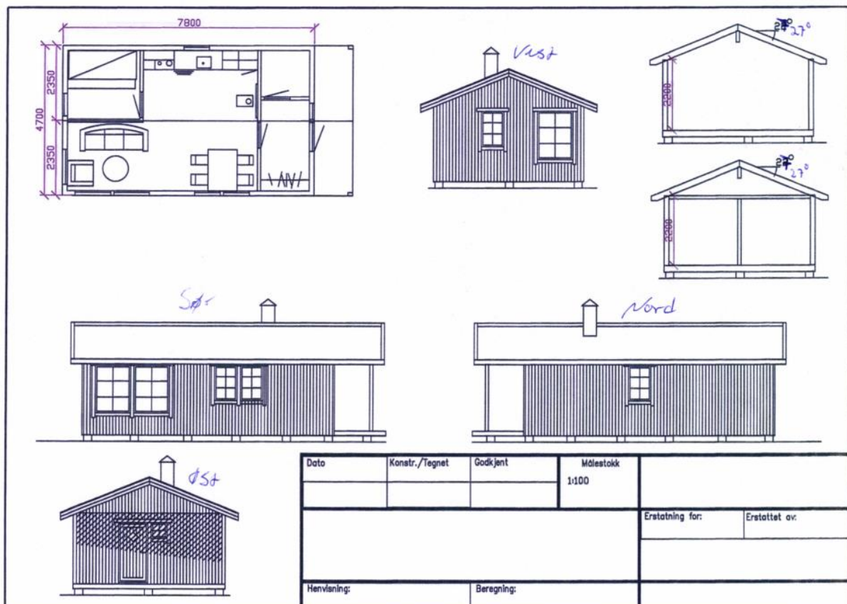
Fig. 1: Tegninger over omsøkt gjeterhytta ved Hykla, sommerboplassen til Låarte sijte i Lierne kommune.
