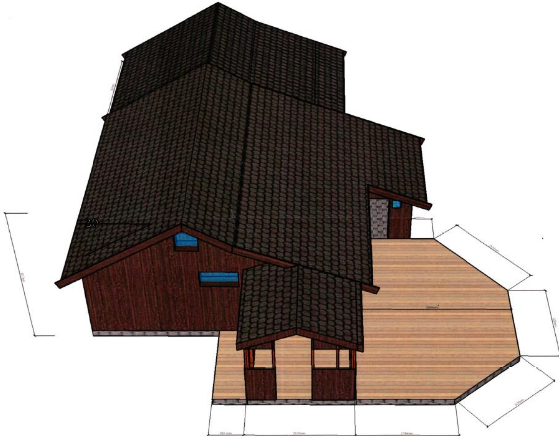
Fig. 1: Målsatt tegning over omsøkte nordvestvendt platting ved hytte Skjækervatnet 32 med Gnr/Bnr/Fnr 80/1/8 i Snåsa kommune.
