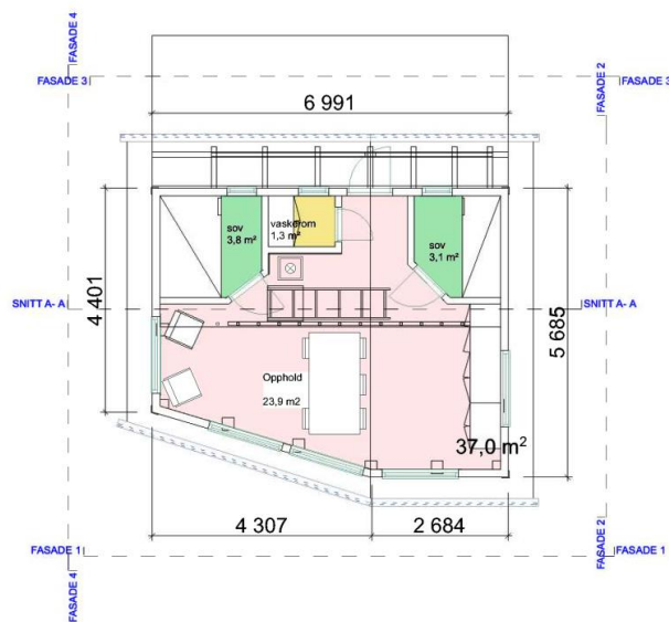
Fig. 1: Byggetegninger datert 23. september 2016 hentet fra søknaden fra Snåsa fjellstyre.
