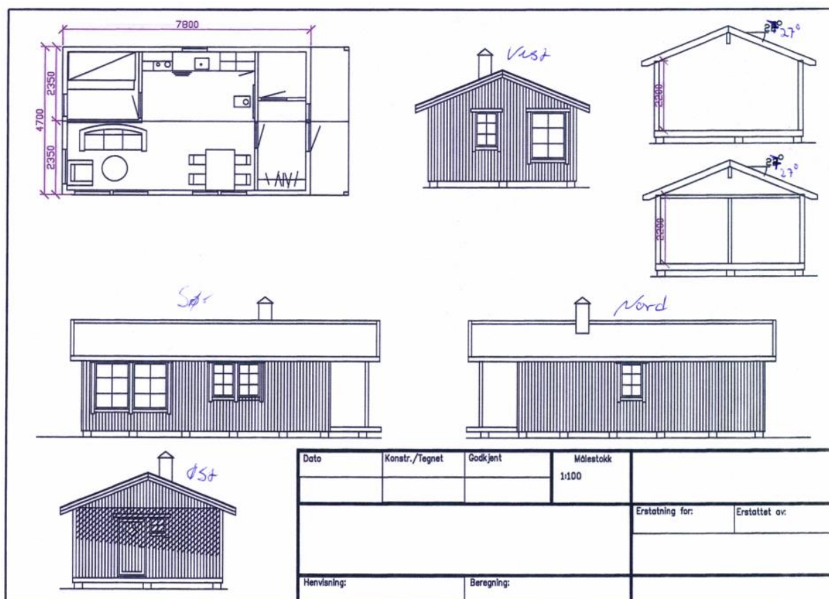
Fig. 1: Tegninger over omsøkt gjetterhytte ved Hykla, sommerboplassen til Låarte sijte i Lierne kommune.
