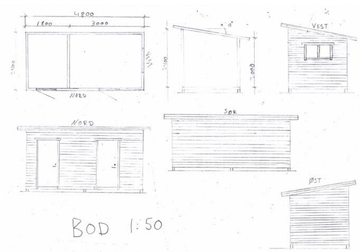
Fig. 1: Tegninger over omsøkt uthus til gjetterhytte ved Hykla, sommerboplassen til Låarte sijte i Lierne kommune.
