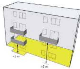
Figur 2-7 Utkragede bygningsdeler medregnes i bebygd areal når høyden til planert terreng er mindre enn 0,5 m.
