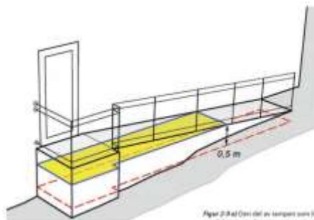
Figur 2-9 a) Den del av bygningen som ligger høyere enn 0,5 m over planert terrengs gjennomsnittsnivå rundt bygningen medregnes i bebygd areal.
