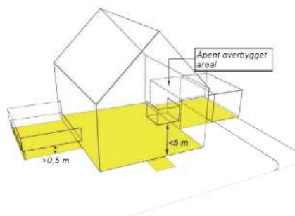
Figur 2-3 Bebyggingsareal (BYA) for bygning
