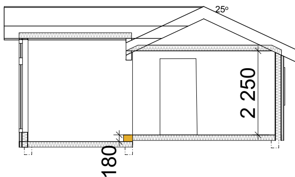
Snitt A
