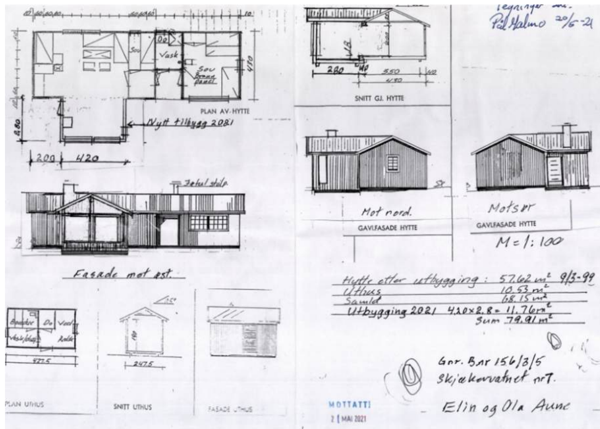
Fig. 1: Tegninger av Skjækervatnet 7, Gnr/Bnr/Fnr 156/3/5
