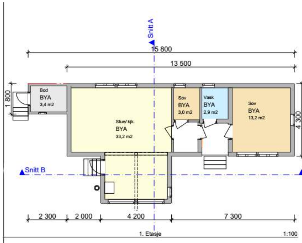
Figur 3: Nye tegninger av hytta, inkl. utedo/bod.
