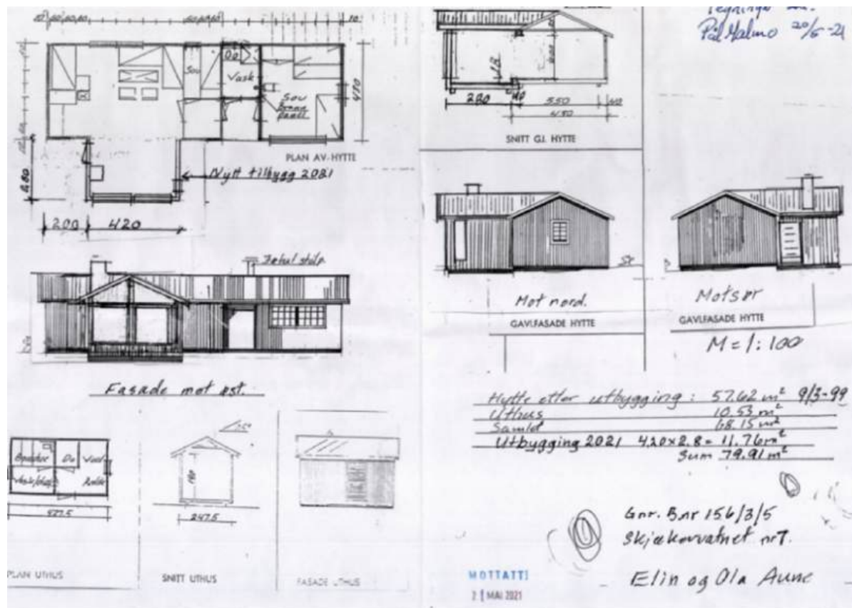
Figur 1: Tegning/skisse som var vedlagt dispensasjonssøknad i 2021.
