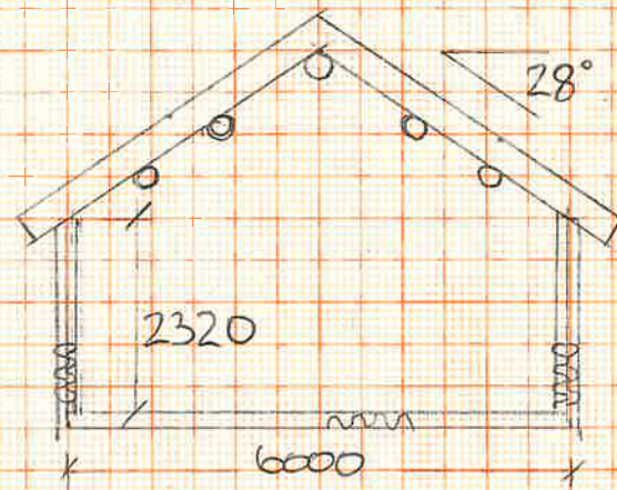
Snitt hytte
